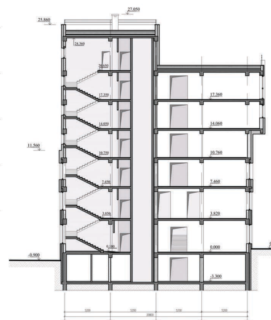
Разрез 1-1
