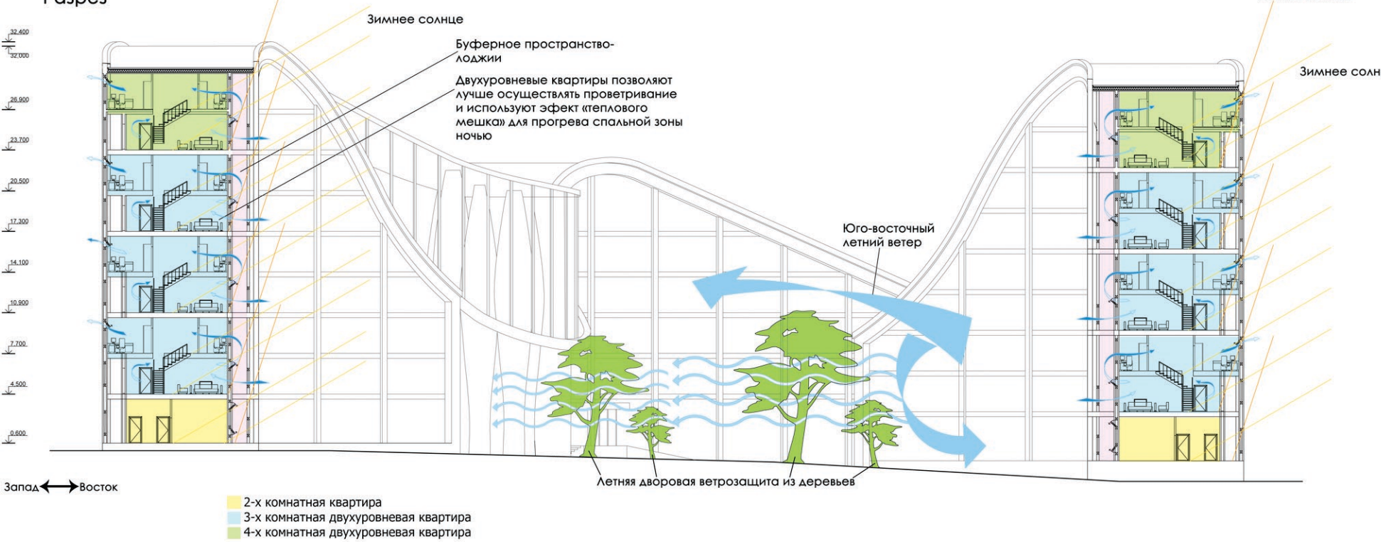
Разрез
