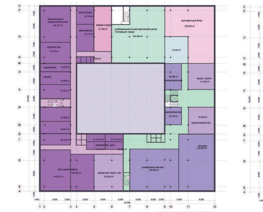
СХЕМА ПЛАНА 1 ЭТАЖА
