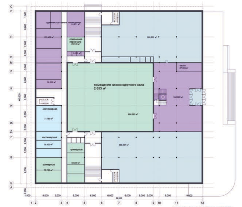
СХЕМА ПЛАНА ЦОКОЛЬНОГО ЭТАЖА
