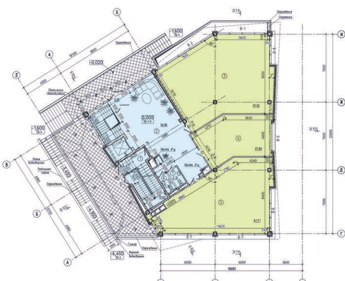
План подвального этажа на отм. 0,000
