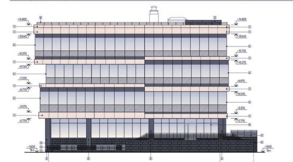
Фасад в осях Г-И
