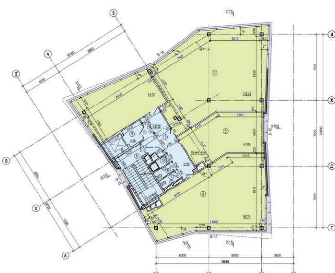
План типового этажа
