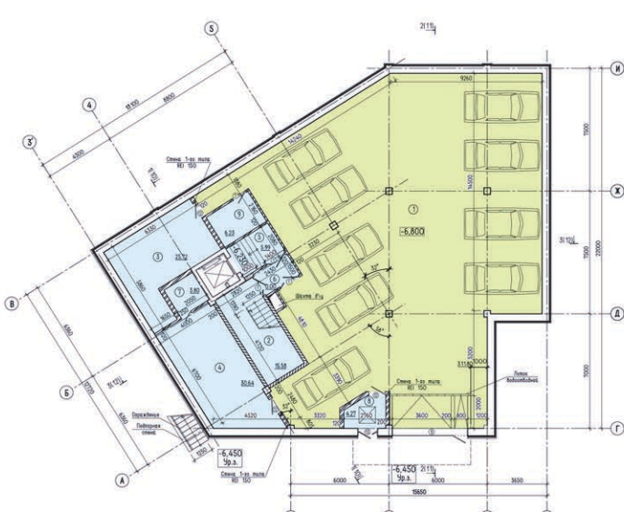
План подвального этажа на отм. -6,800
