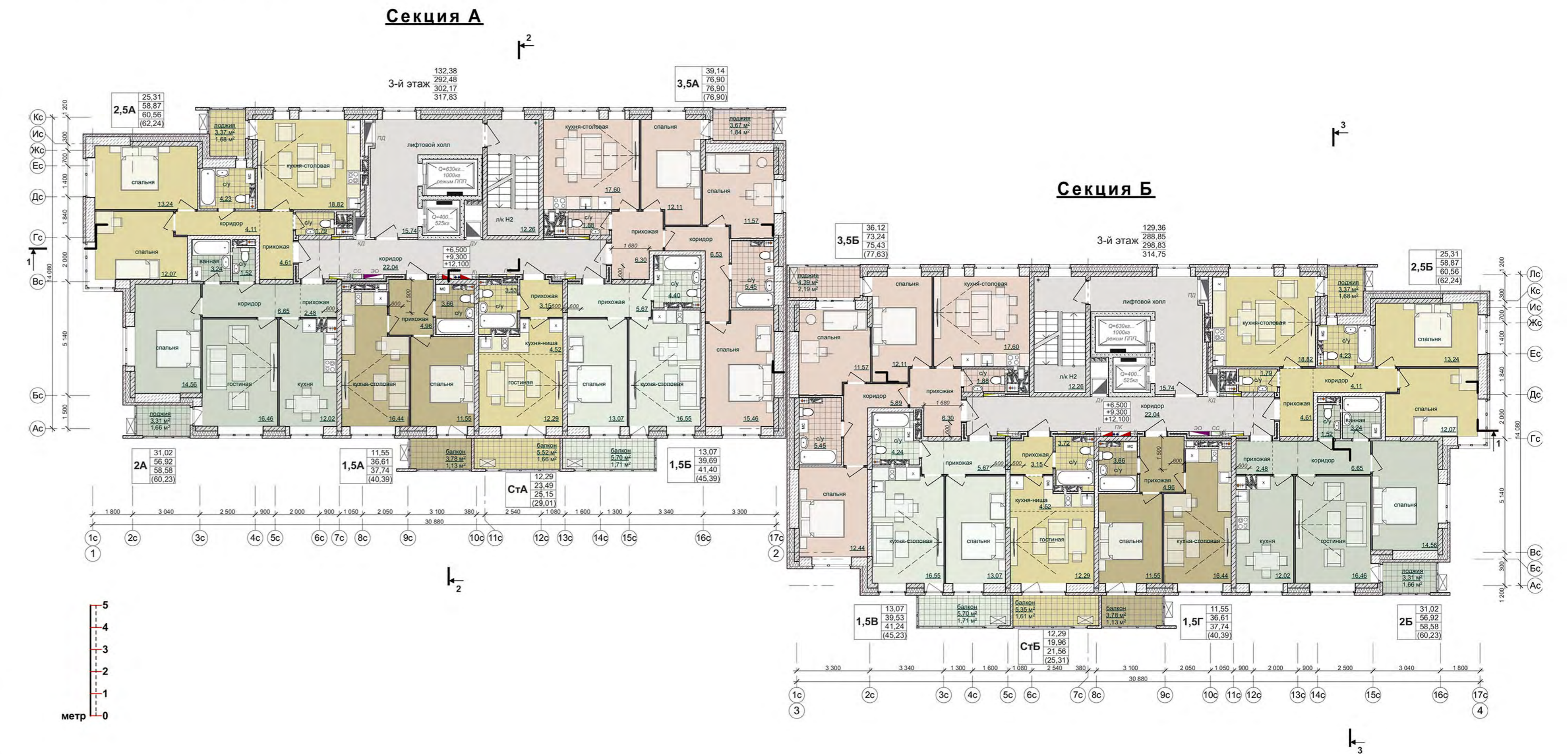
ПЛАН ТИПОВОГО ЭТАЖА
