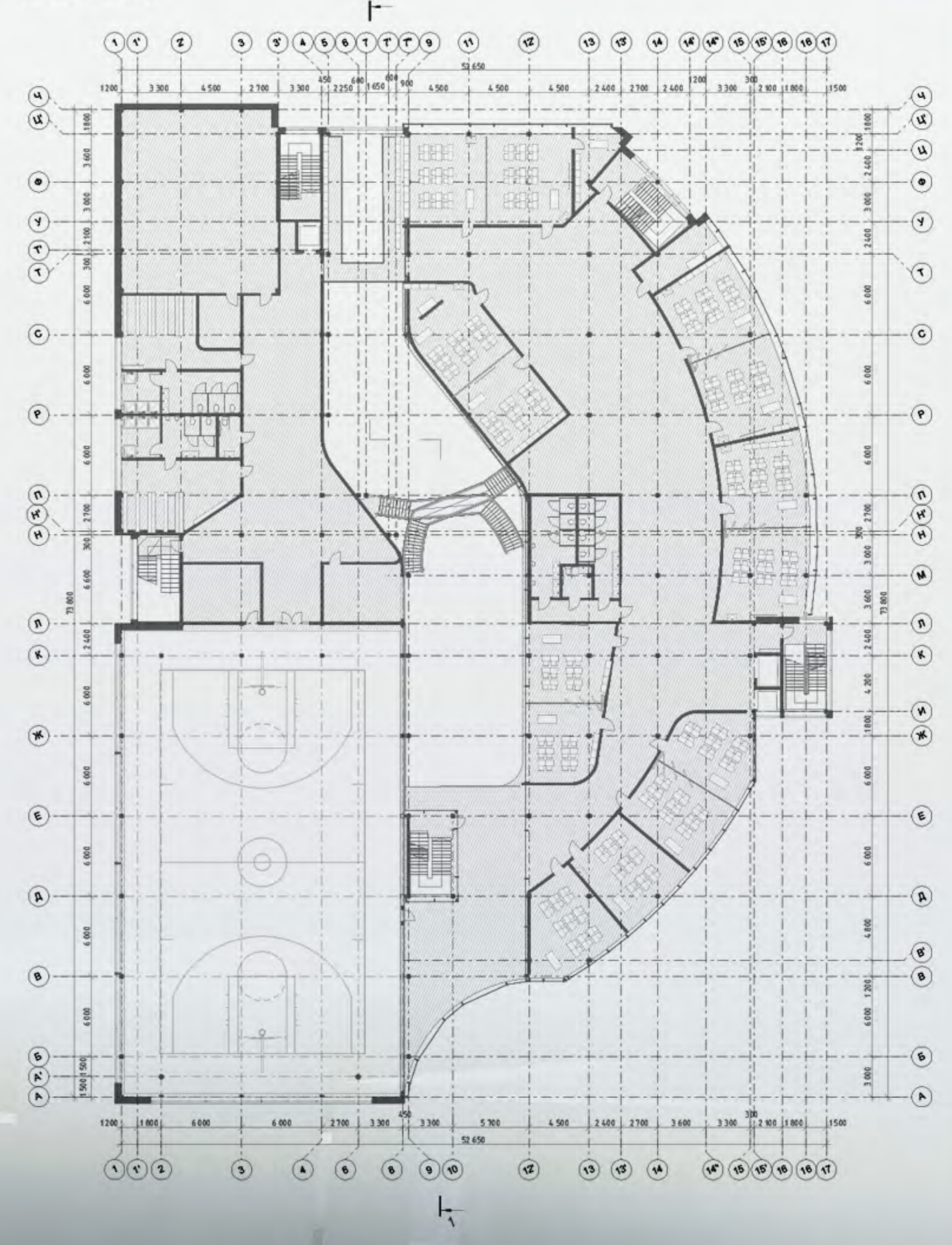
План 2 этажа
