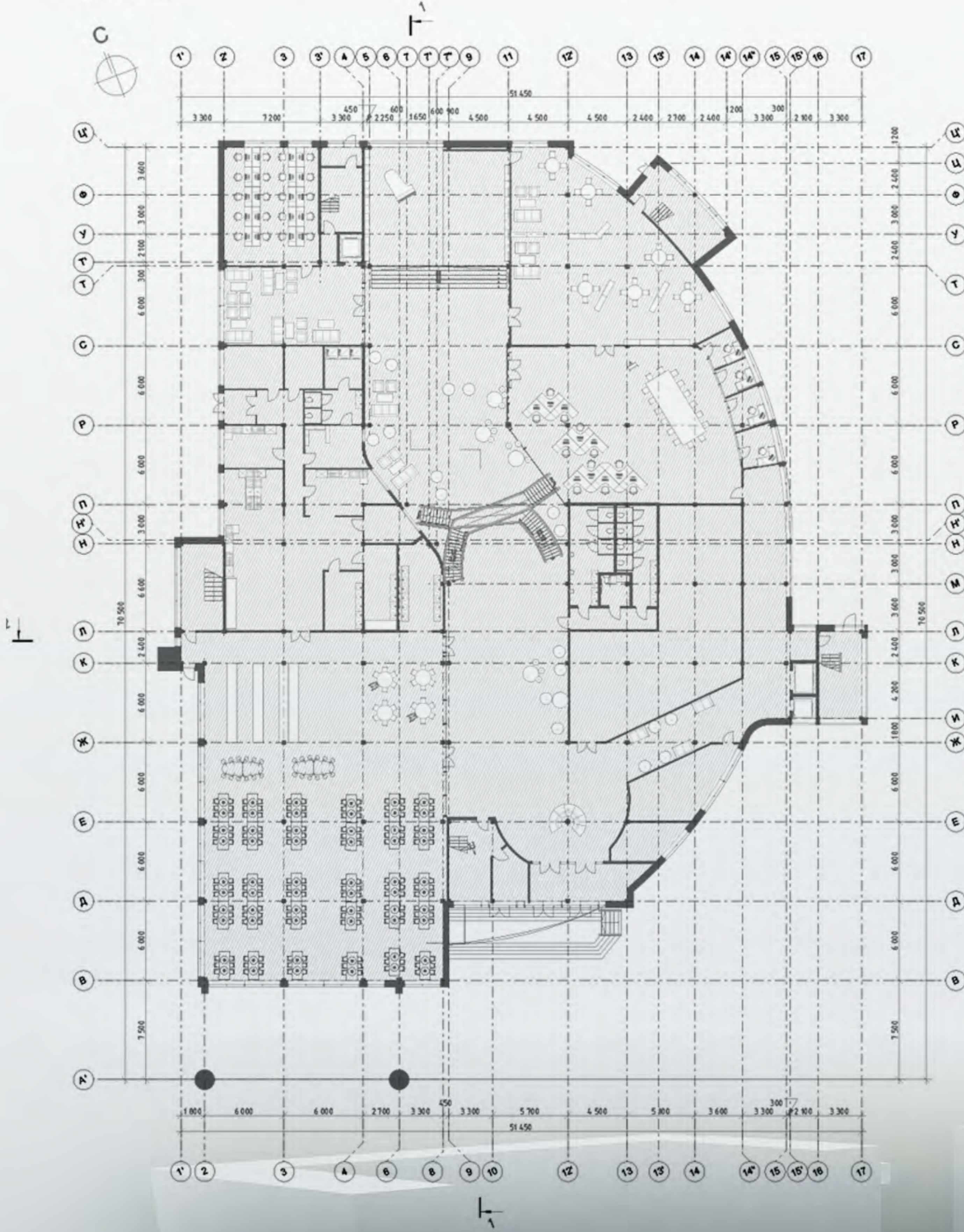
План 1 этажа
