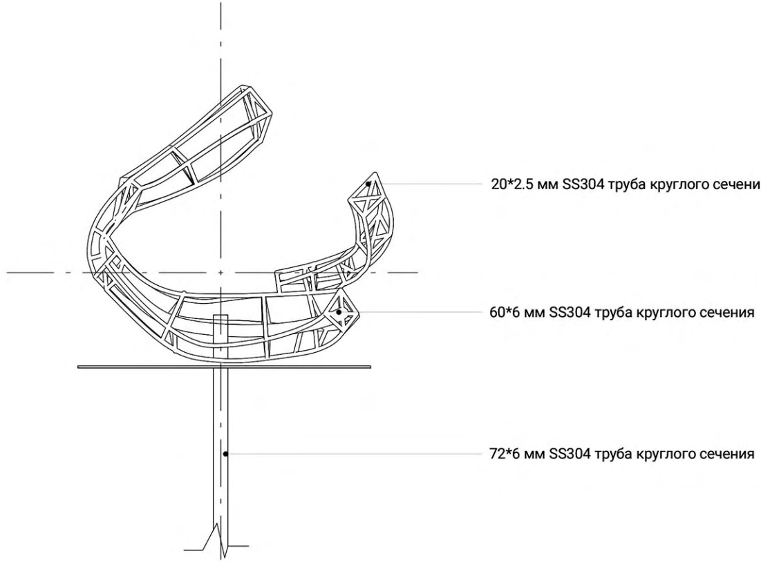
Детализированный чертеж усиления каркаса
