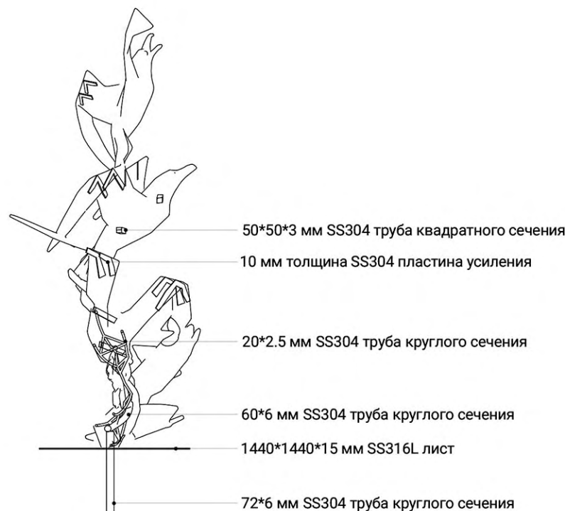
Вид сбоку
